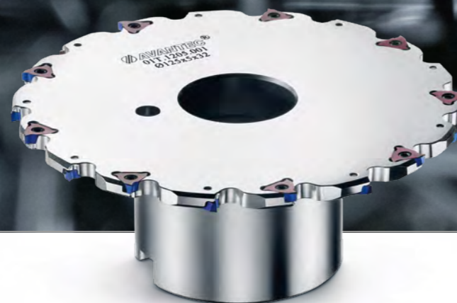
Scheibenfräser TB18
